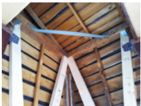
・火打金物で補強
